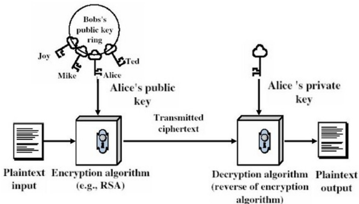
Schema di funzionamento della crittografia a chiave pubblica
